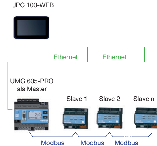
Abb.7: Bus-Topologie mit einem UMG 605 als Master und angeschlossenen JPC 100-WEB
