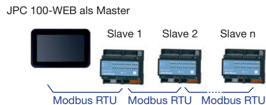
Abb.8: Bus-Topologie mit dem JPC 100-WEB als Master
