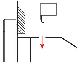
Abb.3: Halteklammern einsetzen.
