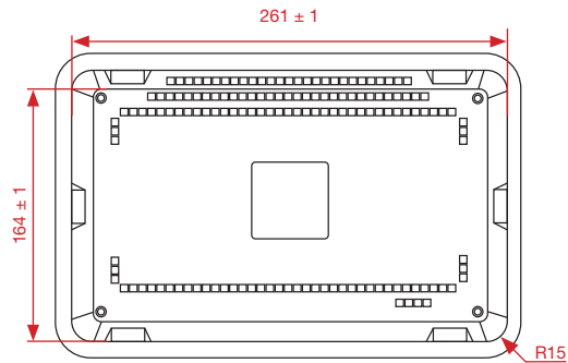
Abb.1: Einbaulage des JPC 100-WEB
