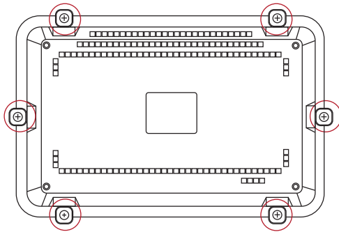
Abb.2: Rückansicht mit Halteklammern
