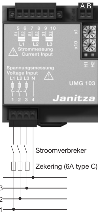
Afb. aansluitvoorbeeld: Spanningsmeting via stroomverbreker en zekeringen.
