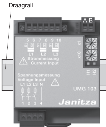
Afb. UMG103 op draagrail conform DIN EN 60715.
