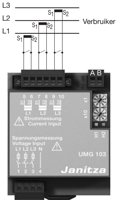
Afb.: Aansluitvoorbeeld, stroommeting via stroomtransformatoren.
