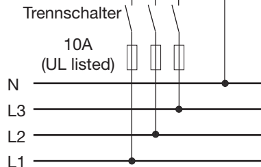
Abb.30.1 Anschlussbeispiel: Spannungsmessung über kurzschlussfeste Messleitungen.
