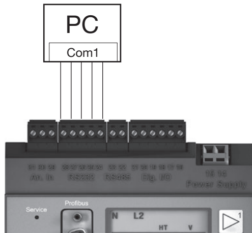
Abb.:33.1 Beispiel, ein UMG104 über die RS232 Schnittstelle mit einem PC verbinden.
