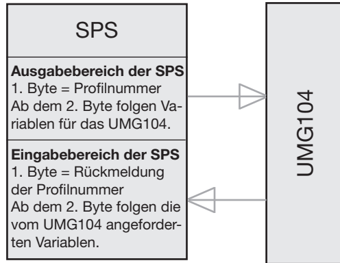
Abb.54.1 Blockschnittbild für den Datenaustausch zwischen SPS und UMG104.
