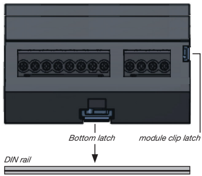
Fig. Device on DIN rail.
